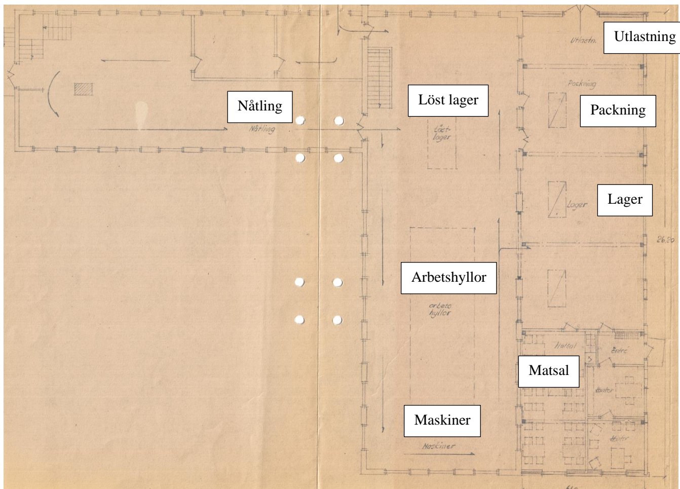
Figur 2. Ritning över förslag till tillbyggnad av skofabriken från 1959.
